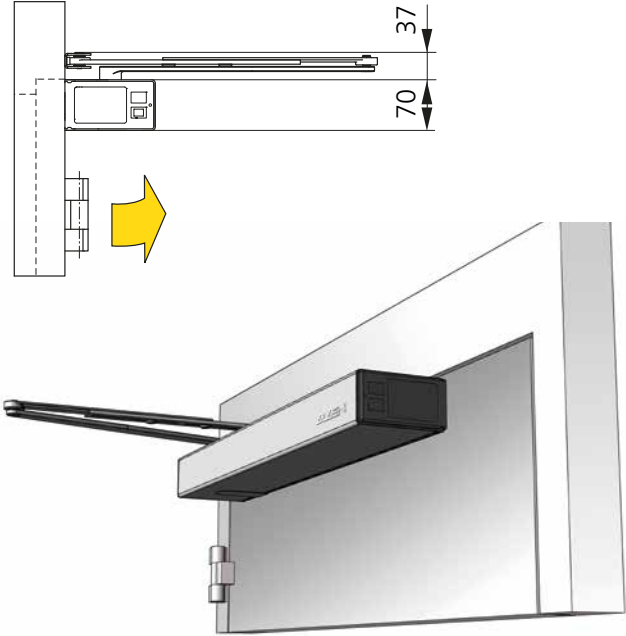
Normalgestänge drückend Flügelmontage
