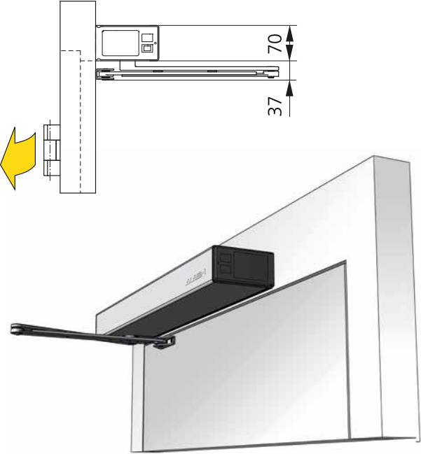
Normalgestänge drückend Sturzmontage
